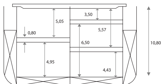
HOLD 1 HOLD 2
